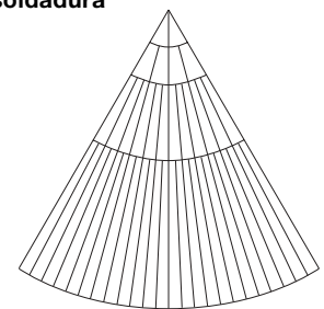
Exemplo de plano de configuração das bandejas e juntas
