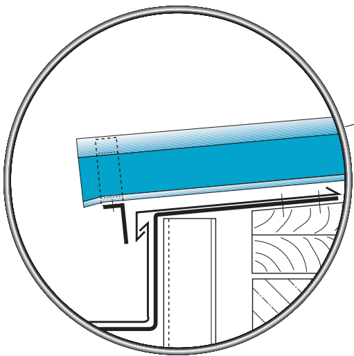
Elemento de estanqueidade fecha o rebordo no beirado
